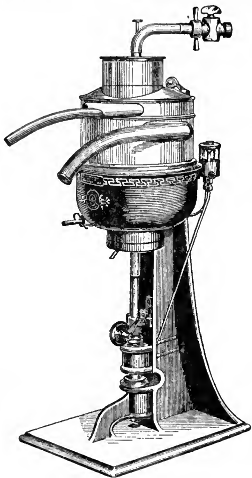
FIG. 19.—Power Separator.
