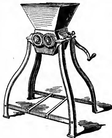
FIG. 6.—Curd-Mill.
