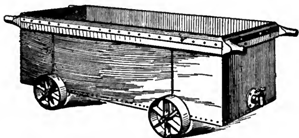
FIG. 3.—Rectangular Cheese-Vat.
