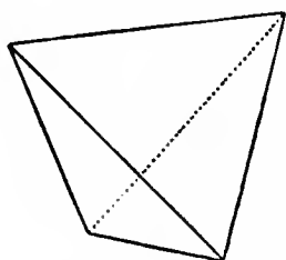
FIG. 26.—Tetrahedron.
