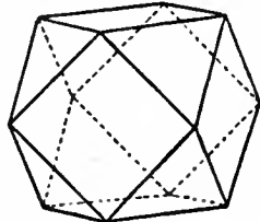
FIG. 7.—Cubo-octahedron.
