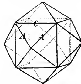
FIG. 22.—Tetrakis-hexahedron.
