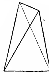
FIG. 61.—Orthorhombic Bisphenoid.
