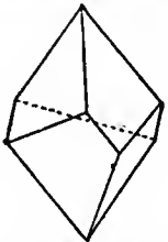
FIG. 74.—Trigonal Trapezohedron.
