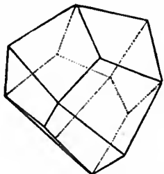
FIG. 27.—Deltoid Dodecahedron.
