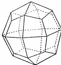
FIG. 17.—Icositetrahedron.
