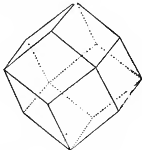
FIG. 13.—Rhombic Dodecahedron.
